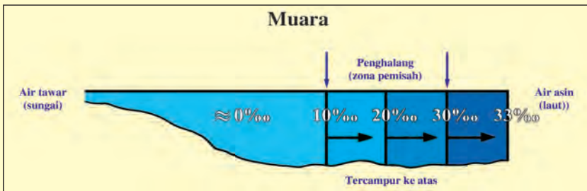
Gambar 14: Penampang panjang yang menggambarkan tingkat keasinan (satu per seribu %) di muara. Di sini terlihat penghalang (zona pemisah) antara air tawar dan air laut. ( Introductory Oceanography [Pengenal terhadap Ilmu kaji Samudera], Thurman, hal. 301, dengan sedikit penajaman).
