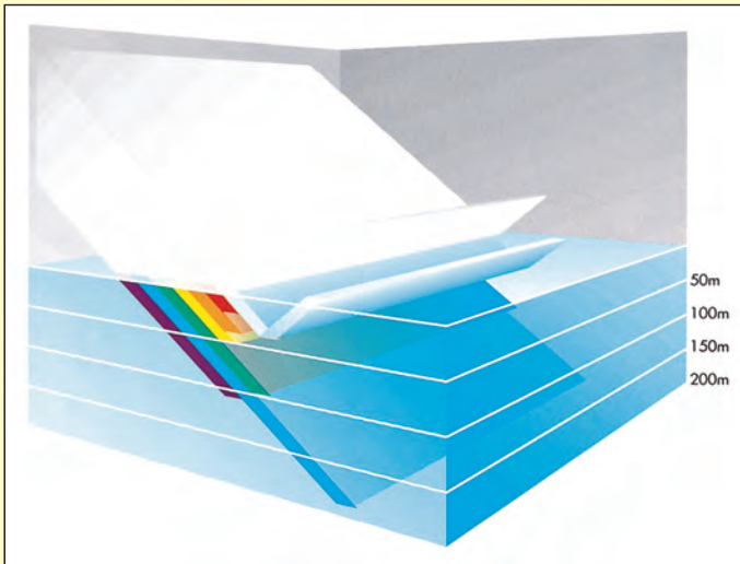
Gambar 15: Antara 3 hingga 30 persen cahaya matahari dibelokkan di permukaan laut. Setelah itu, hampir seluruh ketujuh warna spektrum cahaya diserap satu demi satu pada 200 meter permukaan pertama, kecuali warna biru. ( Oceans [Lautan], Elder dan Pernetta, hal. 27.)
