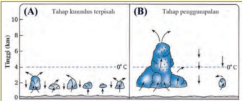
Gambar 19: (A) Serpihan-serpihan awan (awan kumululus). (B) Ketika awan-awan kecil bergabung, gerakan udara vertikal meningkat, sehingga awan pun menggumpal. Butiran air ditunjukkan oleh . ( The Atmosphere [Atmosfera], Anthes et al, hal. 269.)
