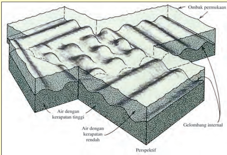
Gambar 16: Gelombang internal pada pertemuan dua lapisan air laut dengan massa jenis yang berbeda. Yang pertama lebih rapat (lapisan bawah), sedang yang kedua kurang rapat (lapisan atas). ( Oceanography [Ilmu kaji Samudera], Gross, hal. 204.)
