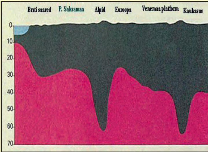
Joonis 8: Skeem mägede ehitusest. (Cailleux. Anatomy of the earth. Lk. 220)
