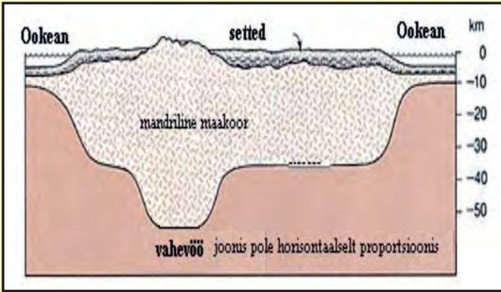
Joonis 7: Mägedel on maa all sügavad juured. (Press & Siever. Earth. Lk. 413)
