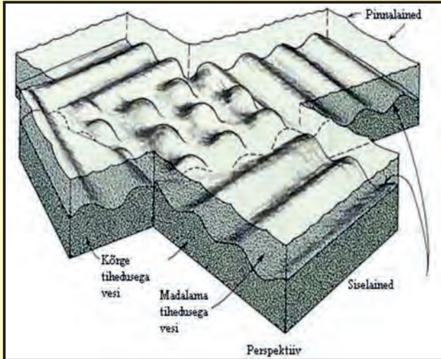
Joonis 16: Siselained kahe erineva tihedusega veekihi vahel. Alumine veekiht on kõrgema tihedusastmega kui ülemine. (Gross. Oceanography. Lk. 204)
