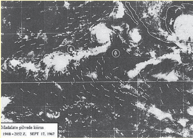
Joonis 17: Pilvede liikumine liitumiskiirkondadesse B, C ja D; satelliidifoto. Nooled näitavad tuule suunda. (Anderson. The use of satellite pictures in weather analysis and forecasting. Lk. 188)
