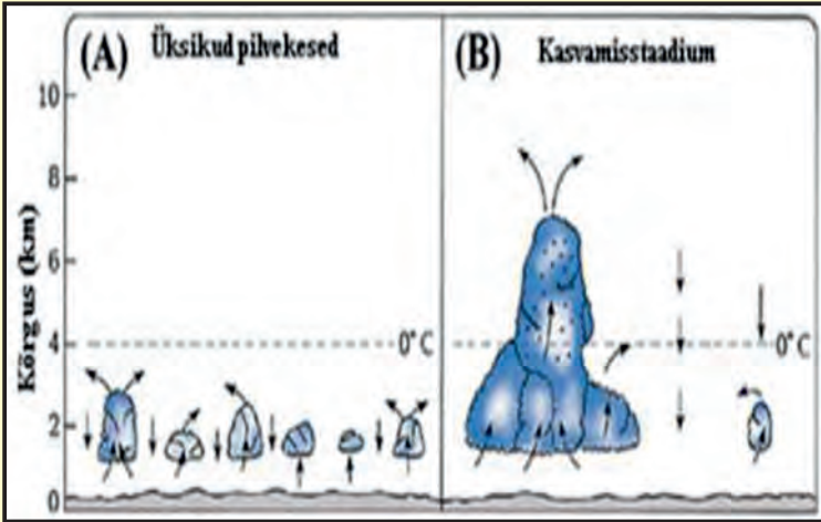
Joonis 19: (A) Üksikud väikesed rünpilved. (B) Kui väikesed pilved on kokku koondunud, moodustab tekkiv ülestõmbejõud vertikaalselt kasvava pilve. (Anthes. The atmosphere. Lk. 269)
